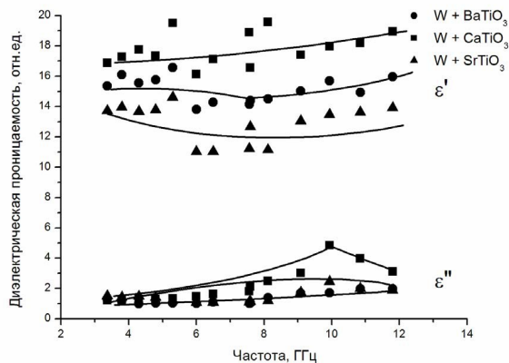
Рисунок 1. Спектры диэлектрической проницаемости смеси BaCo_{0,6}Zn_{1,3}Fe_{16}O_{27}
